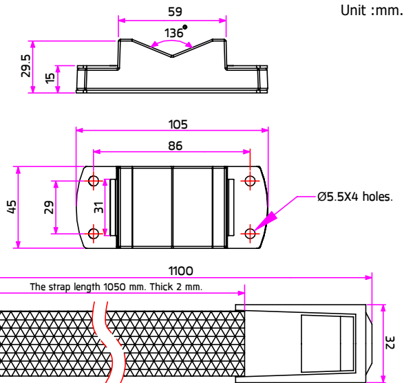
Tree Strap for Small Base / ชุดสายรัดต้นไม้ Ordering Code/รหัสสั่งซื้อ : AUN-TRS-0001-00
